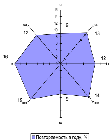
Рис. 1.1.2 Среднегодовая повторяемость (%) направлений ветра по кварталам
